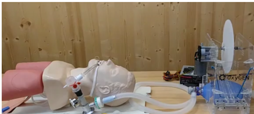
Figura 10. Prototipo de respirador mecánico. (Foto: Oxygen By Ken)
